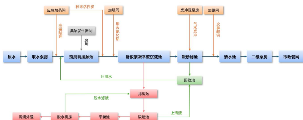
▲ 肖山水厂工艺流程图
