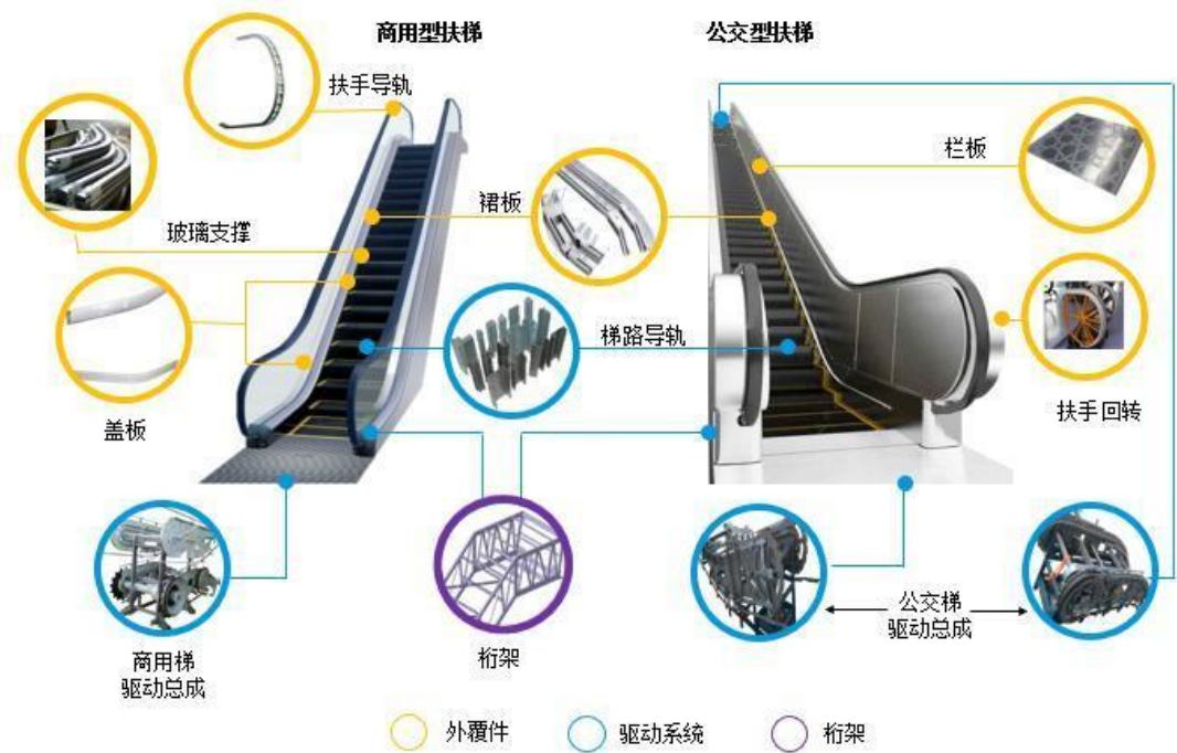
(1) 扶梯主要产品示意图
