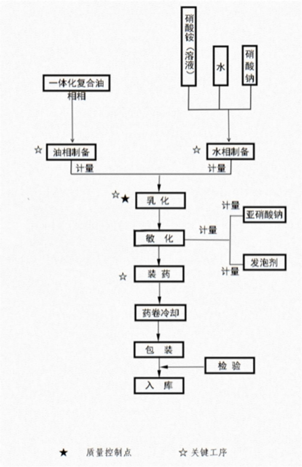
(2) 粉状炸药生产流程
