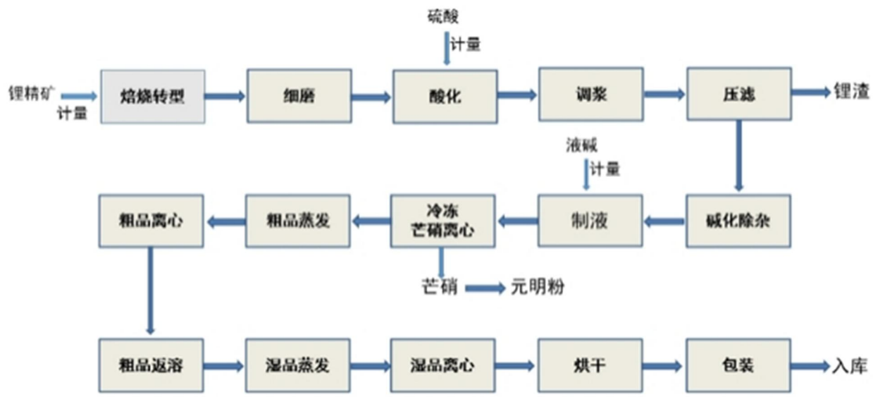
(2) 碳酸锂生产流程
