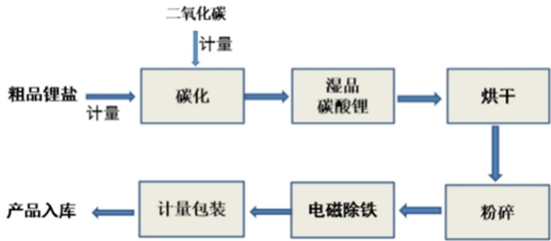
(2) 碳酸锂生产流程
