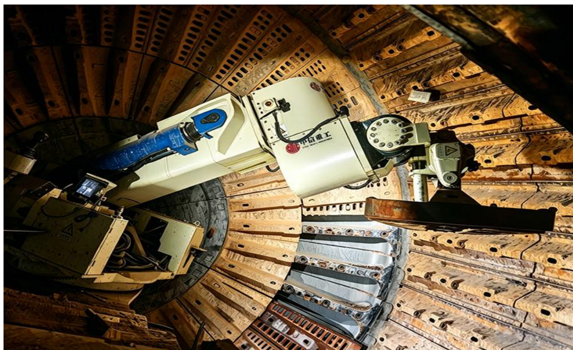
图示：自主研发的七自由度机械手更换矿用磨机耐磨衬板
