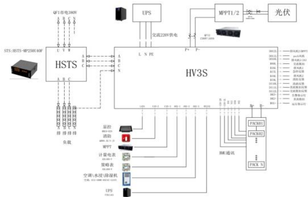
产品拓扑图：
