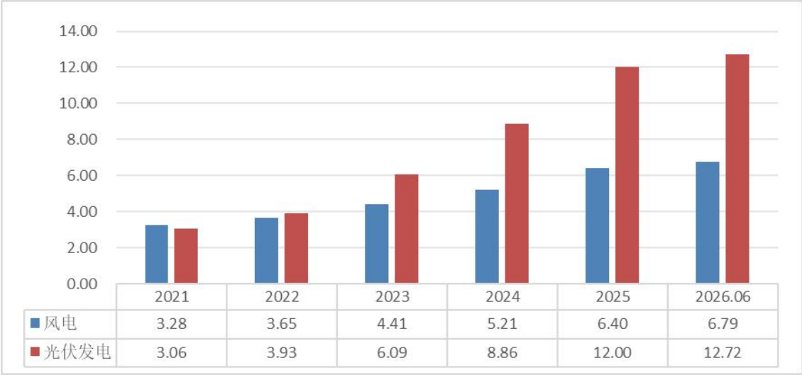
图：近五年全国风电、光伏发电累计装机容量（亿千瓦）
