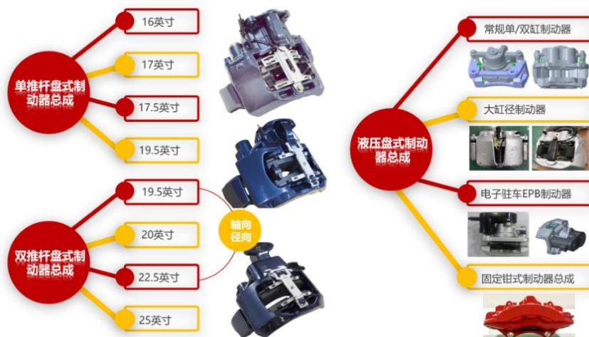
盘式制动器总成
