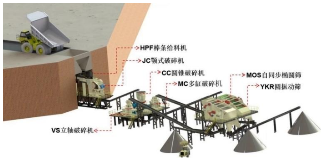
图 9：成套破碎设备生产线示意图
