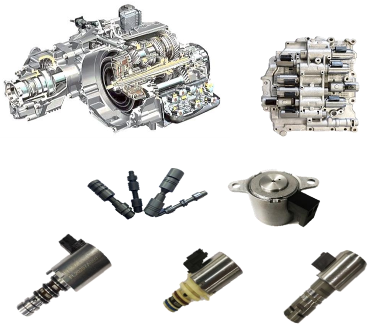
用于 AT & DCT & CVT 电液控制模块的精密电磁阀及阀芯
