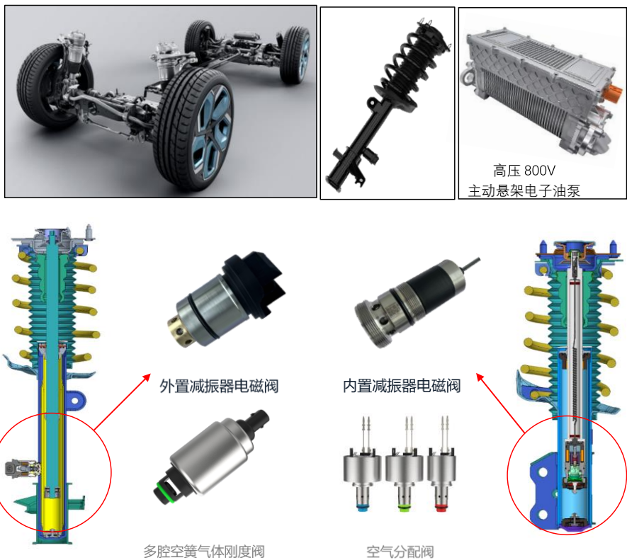
图五：悬架系统零部件
