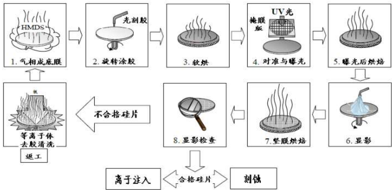
（半导体光刻胶工艺流程示意图）
