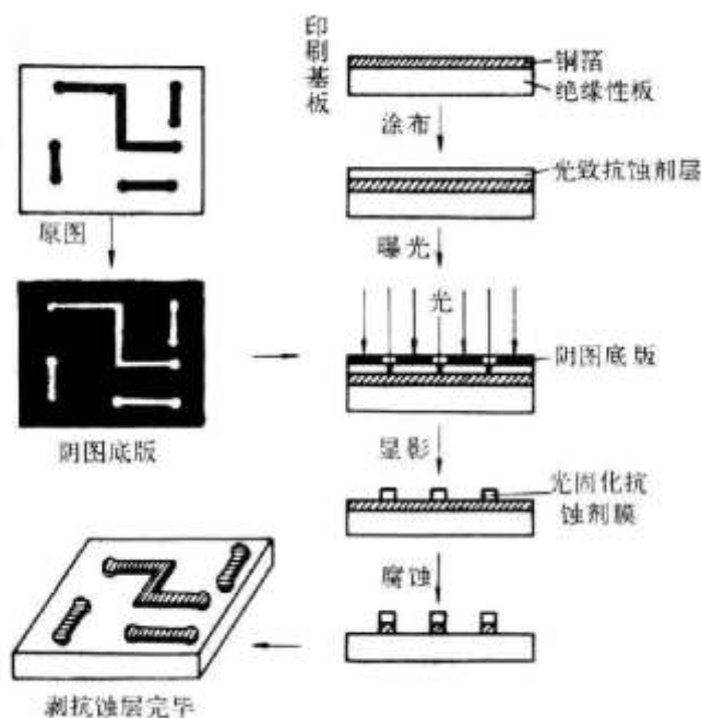
(PCB 光刻胶作用原理示意图)
