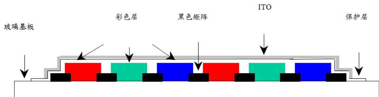
图例：彩色滤光片（ColorFilter）结构简图
